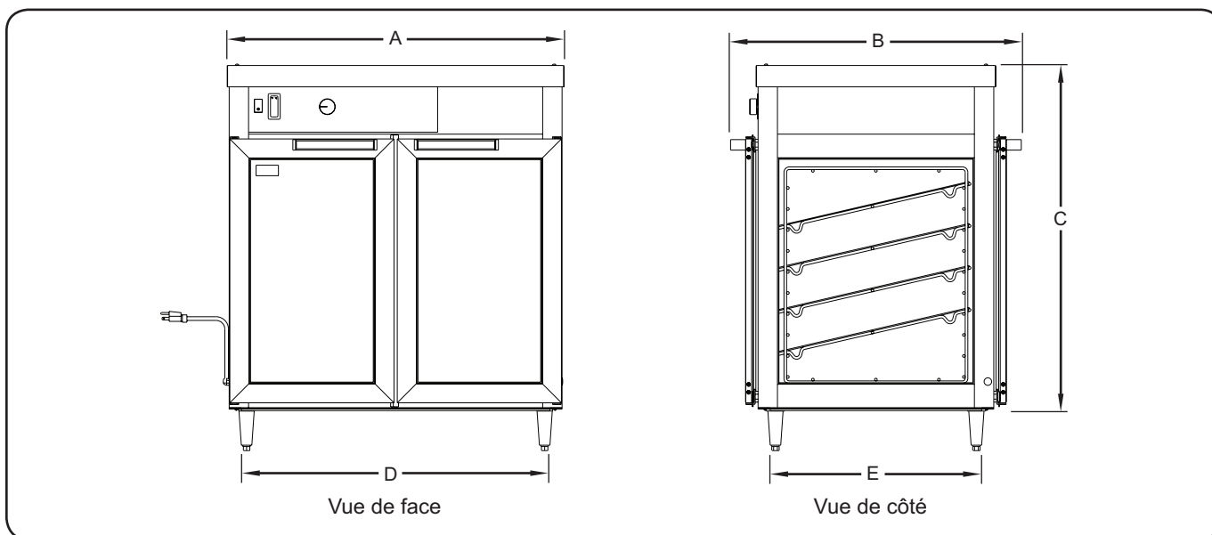
Dimensions du WFST-2X
