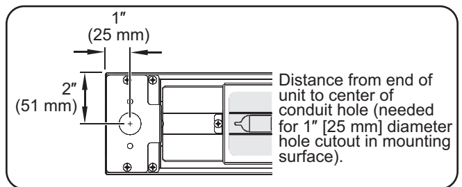
Countertop Conduit Hole Dimension
