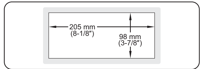
Dimensions pour la découpe du boîtier de commande
