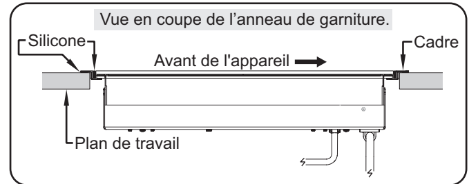
Installation standard avec cadre
