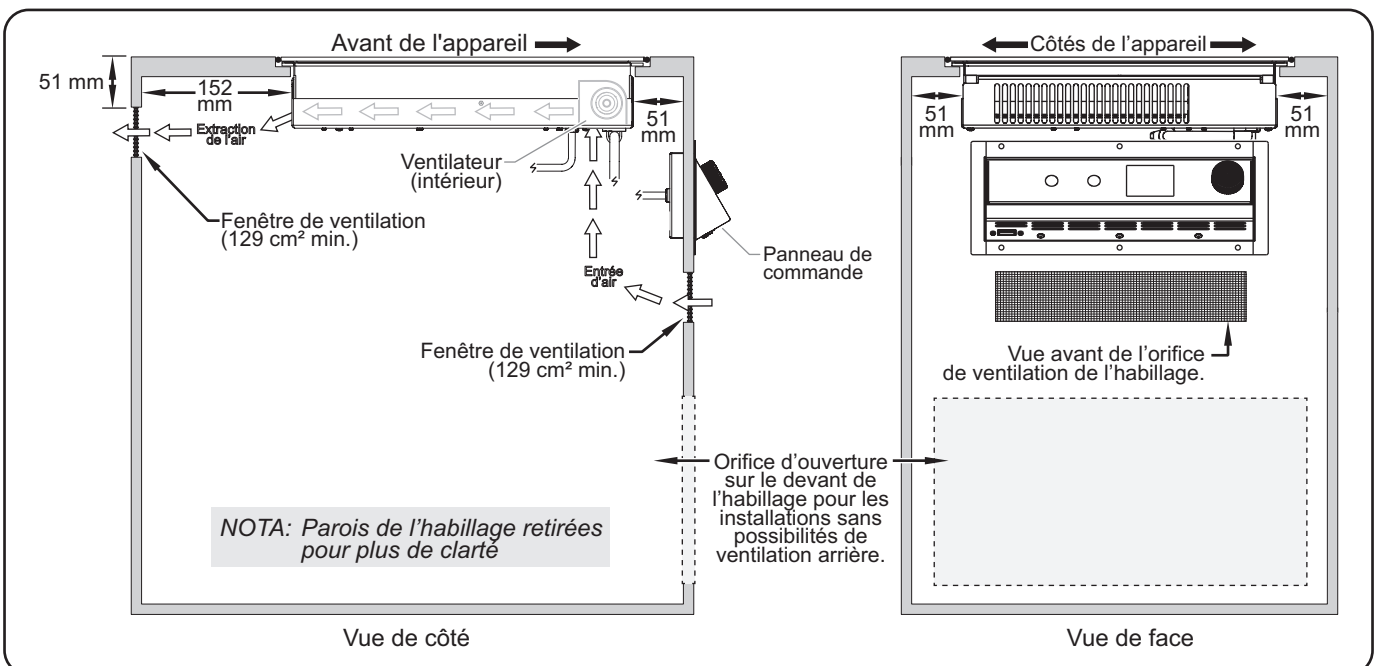
Distances minimales de montage pour les modèles à encastrer
