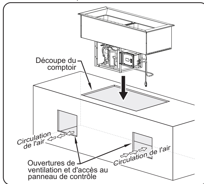
Installation d'un modèle CWB-S2
