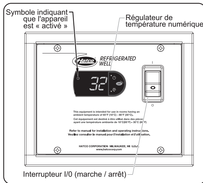
Panneau de contrôle des séries CWB-S
