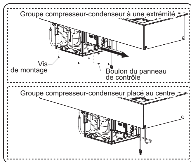
Déplacement d'un groupe compresseur-condenseur
