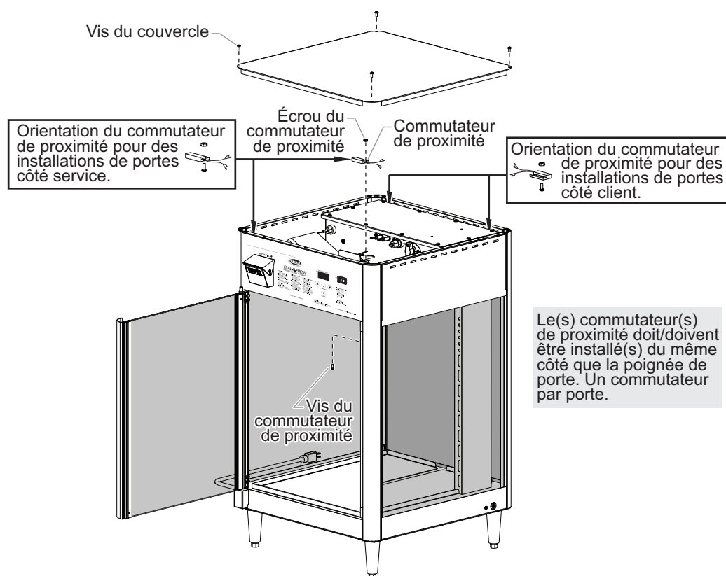
Déplacement du Commutateur de Proximité
