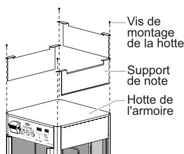
Installation du support d'enseigne de présentoir
