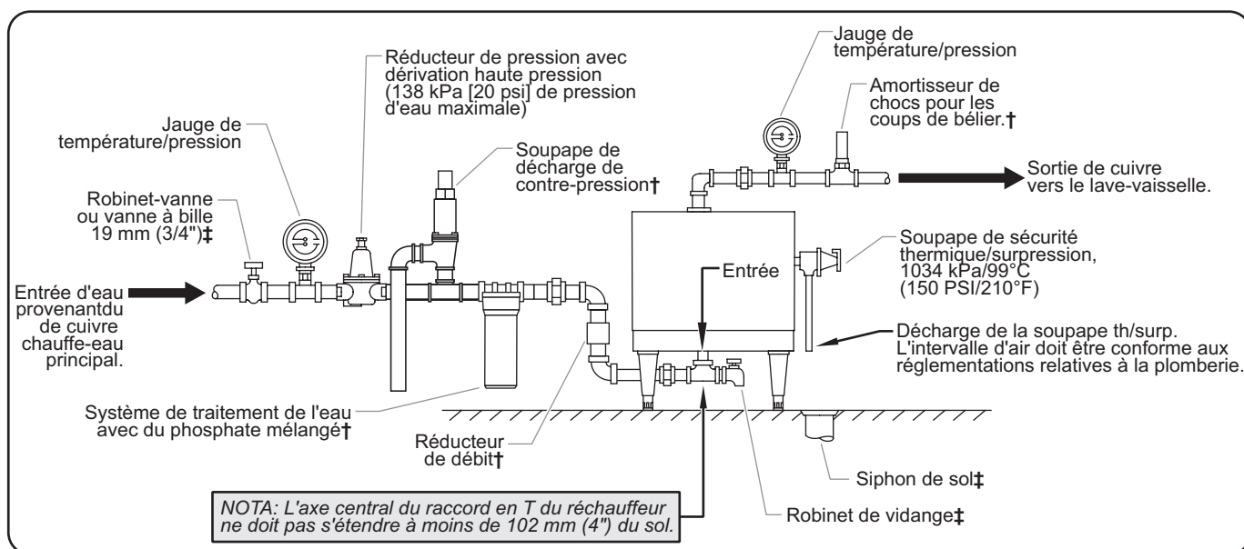
Série « MC » modèles Mini-Compact
