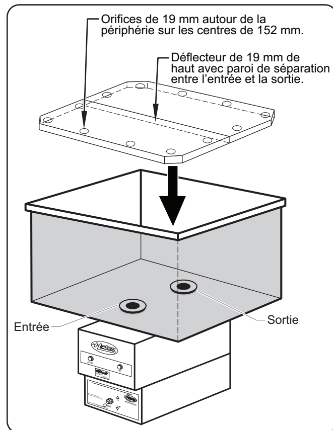
Installation du déflecteur d'eau (Modèles français)
