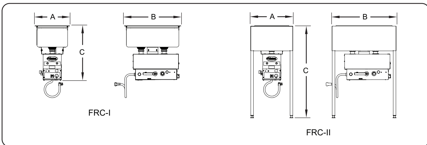
Dimensions—Modèles FRC
