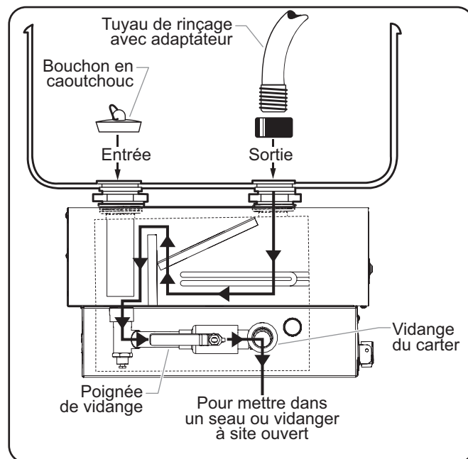
Vidange du réservoir
