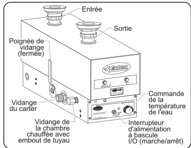
Modèle FR
