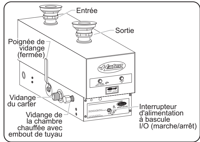
Modèle 3CS
