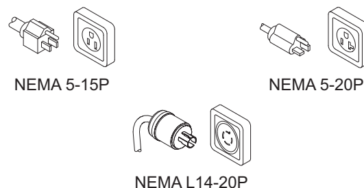
Configuration des fiches
