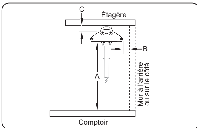
Exigences de dégagement minimum
