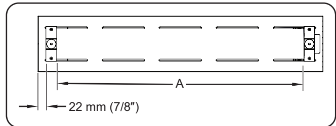
Distances des supports de montage
