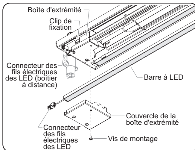
Remplacer un tube d'éclairage
