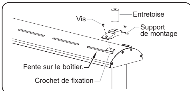
Fixation du support de montage
