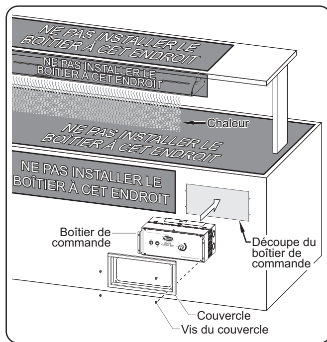
Installation du boîtier de commande GR5AL
