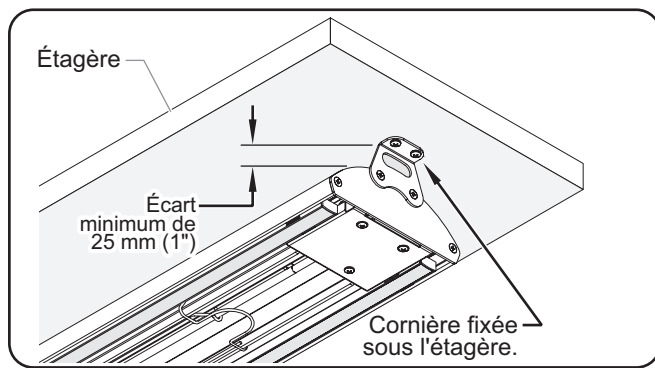
Installation d'une étagère plate
