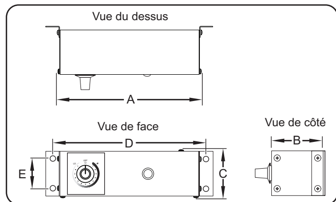
Dimensions du boîtier de commande
