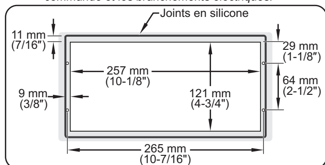
Dimensions de découpe et de passage du boîtier de commande
