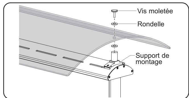
Fixation du pare-haleine
