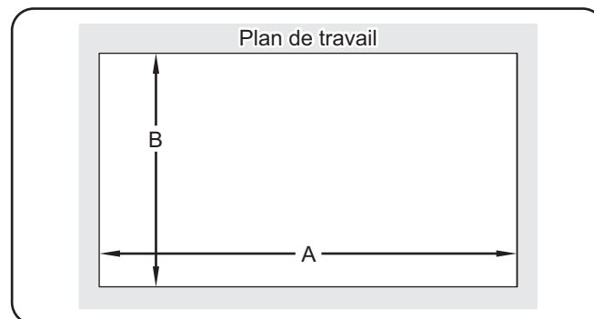
Dimensions de découpe du comptoir
