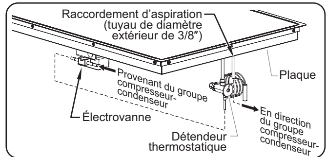
Raccordements du système réfrigéré contrôlé à distance (modèles CSUX, CSBFX, CSSBX, CSSBFX)
