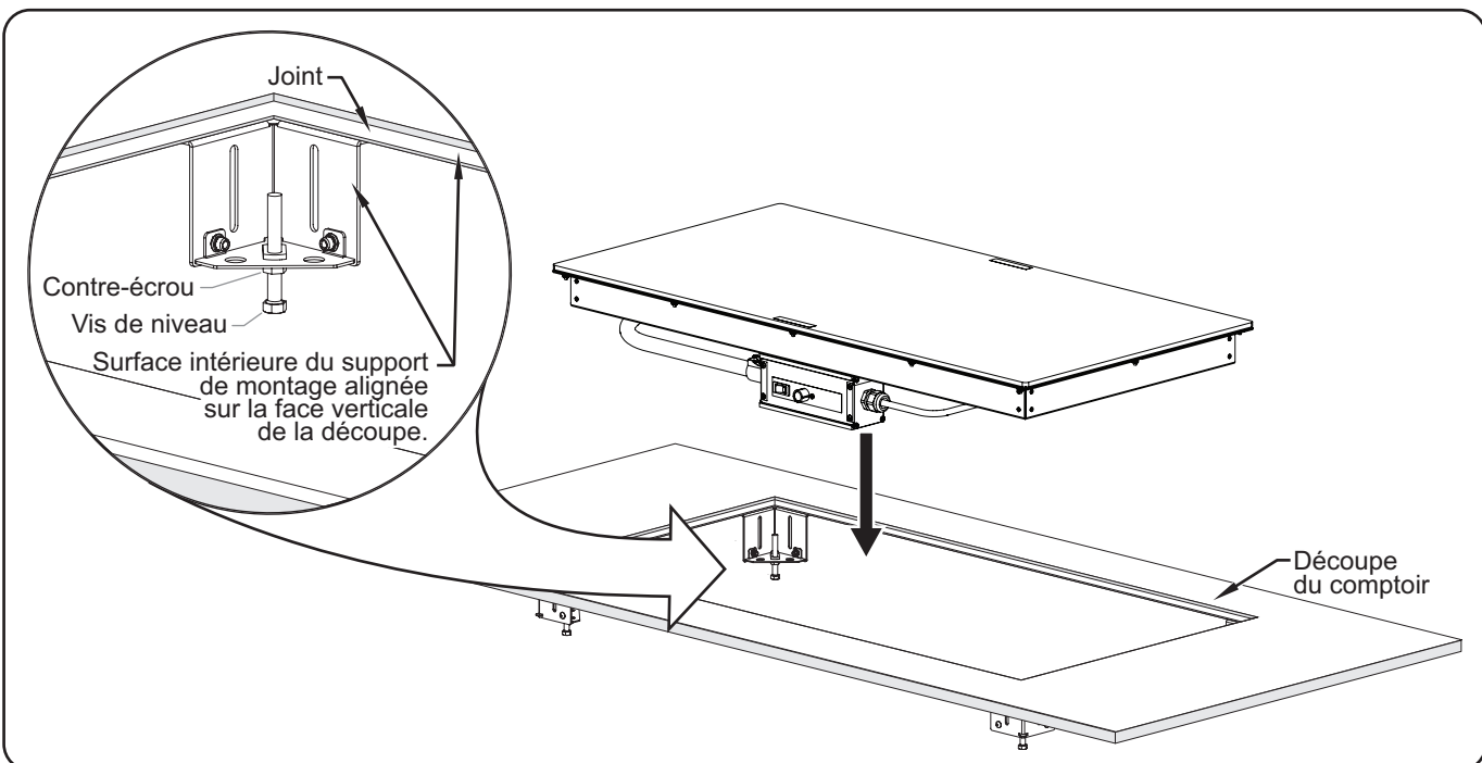
Installation d'une plaque chauffante/réfrigérante modèle HSBF
