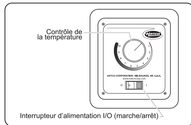
Commande de température mécanique
